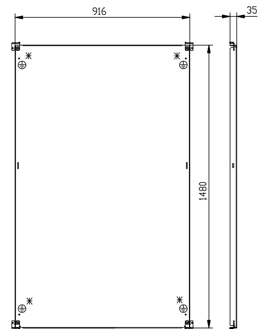
Montageplatte sendzimirverzinkt Blechstärke: 3,0 mm
