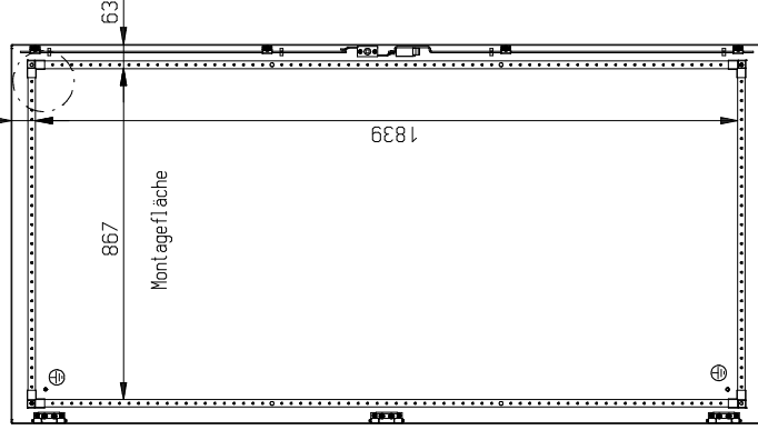
Türe Innenseite
