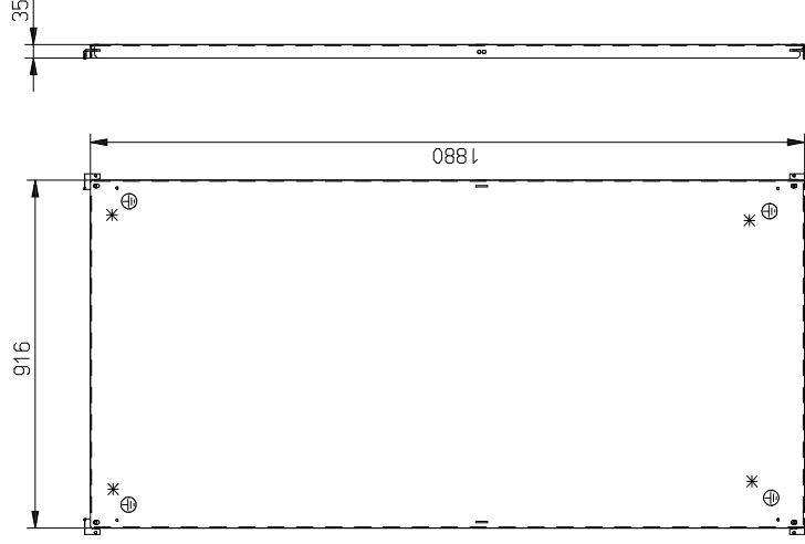
Montageplatte sendzimirverzinkt Blechstärke = 3,0 mm
