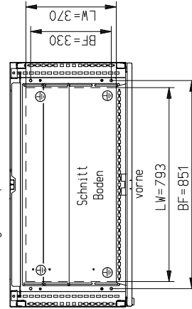
dreiteilige Bodenplatte frei einteilbar
