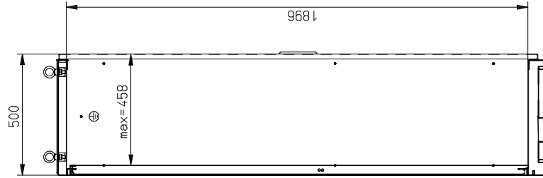
dreiteilige Bodenplatte frei einteilbar
