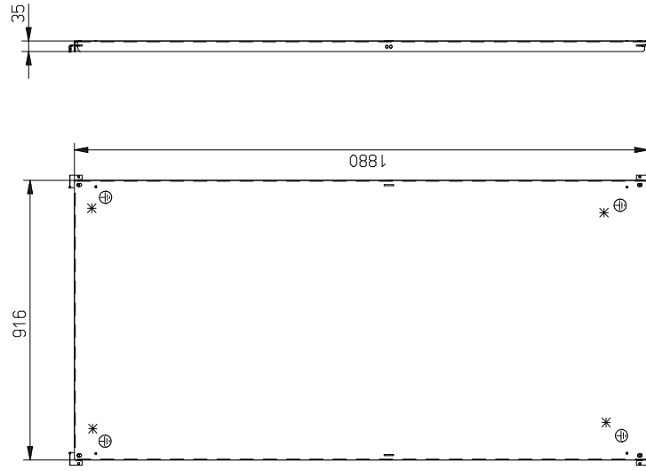
Montageplatte sendzimirverzinkt Blechstärke = 3,0 mm
