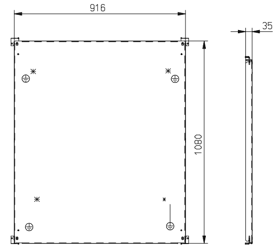
Montageplatte sendzimirverzinkt Blechstärke = 3,0 mm
