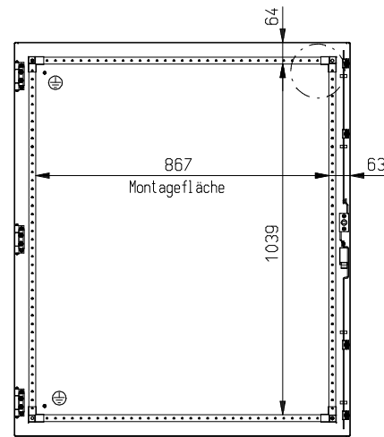
Türe Innenseite
