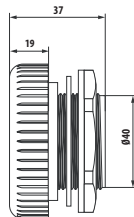
3080-7115-40U15 M40 x 1,5 (IP66/69, IK10) SW50; Ø60
